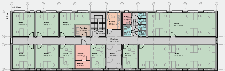
Obergeschoss
