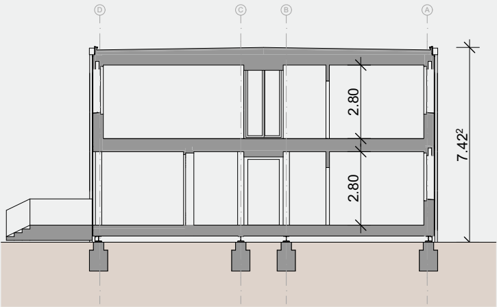
Querschnitt
