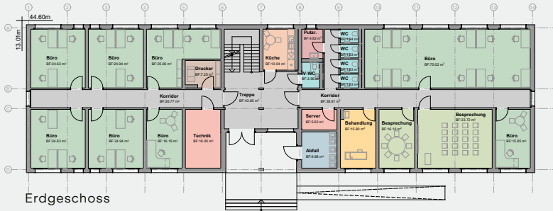
Erdgeschoss
