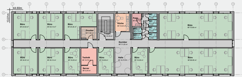
Étage supérieur
