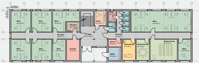
Rez-de-chaussée
