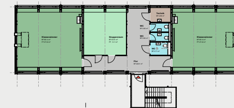
Grundriss Geschoss
