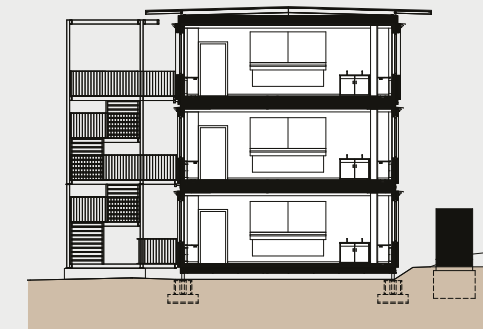
Beispiel Querschnitt dreigeschossiger Bau
