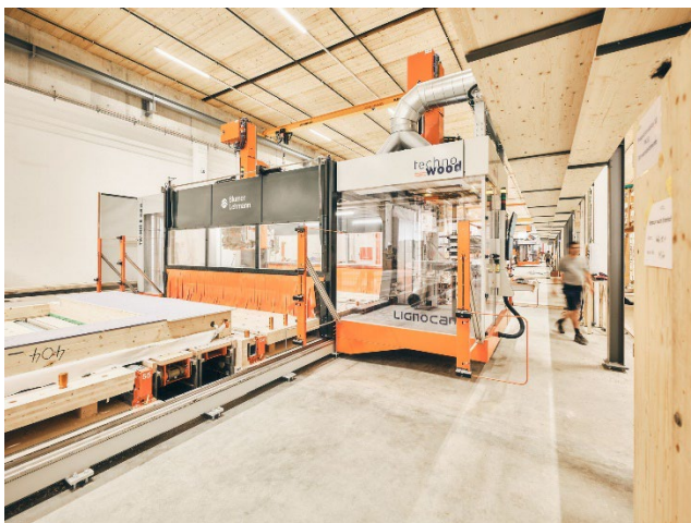
Produktionsstraße für Holzmodulbauelemente (Werk Gossau SG) © Blumer Lehmann
