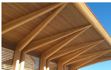
Detailansicht Dachkonstruktion
