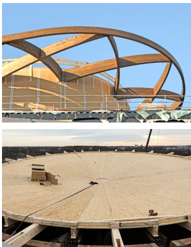
Detailansicht der Dachkonstruktion während den Bauarbeiten
